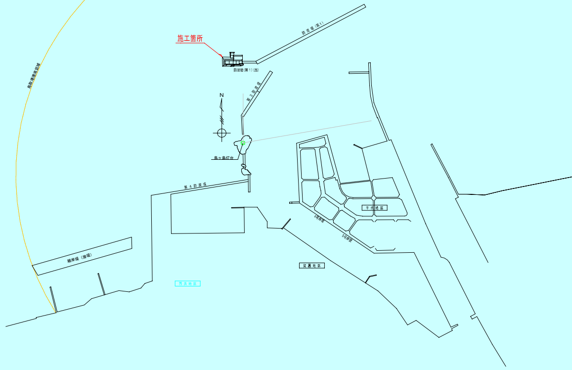
平面図
