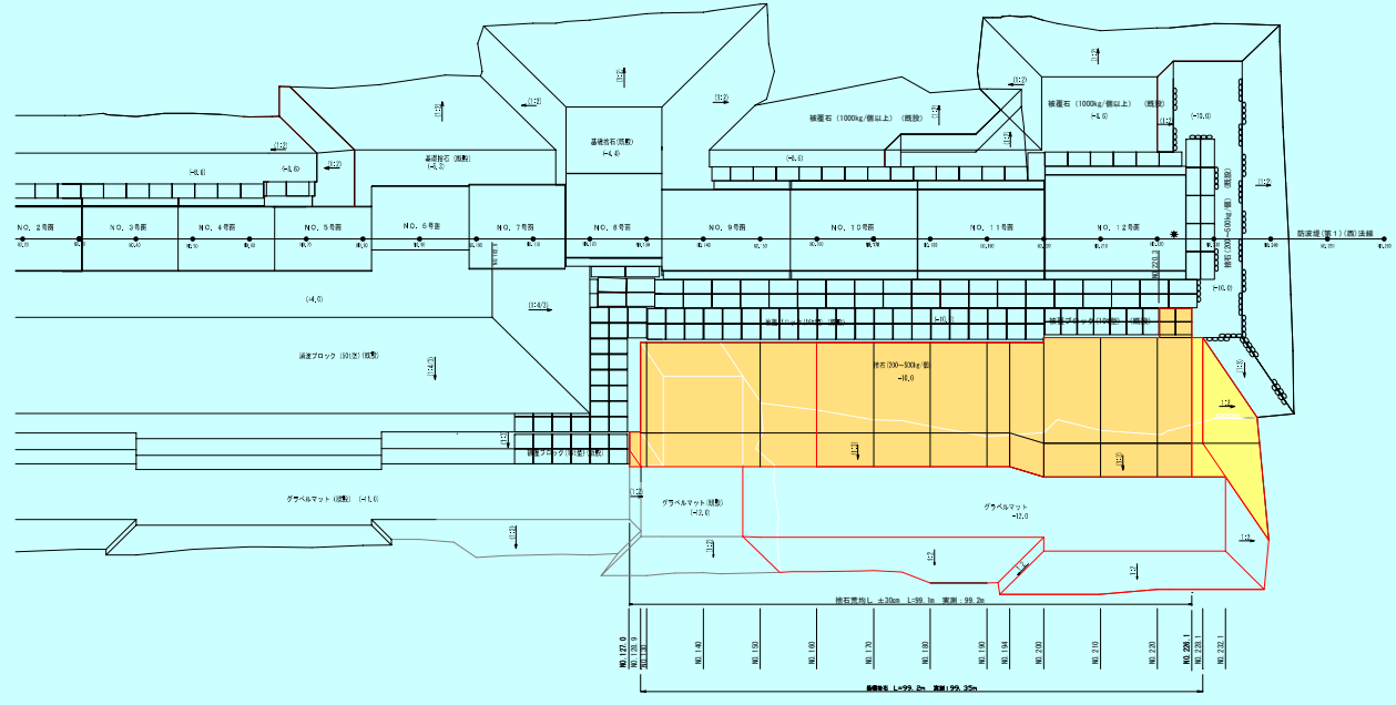
平面図
