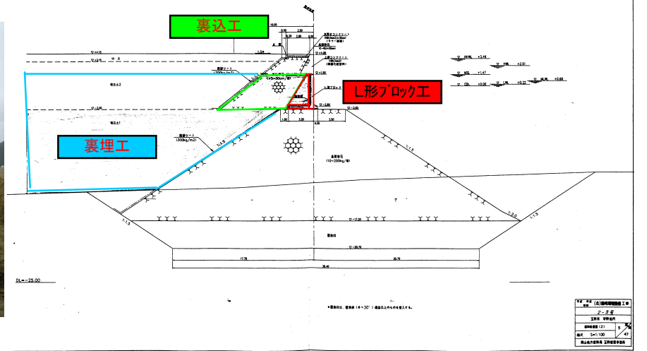
標準断面図 A-A
